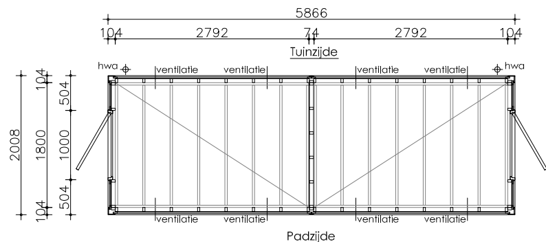
Dubbele berging Type LSPDB: • Aantal getekend : 00 stuks
