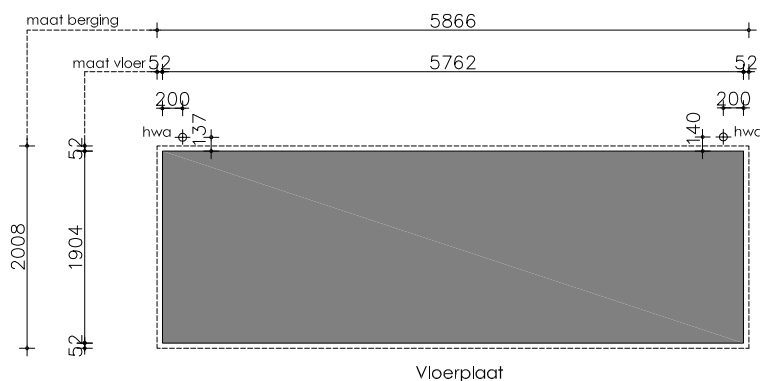
Vloerplaat
