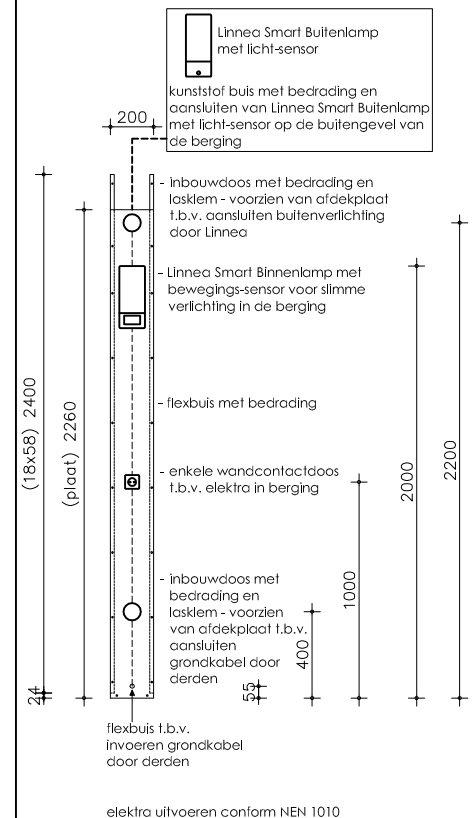
Linnea Smart Installatiepaneel binnenlamp met bewegings-sensor
