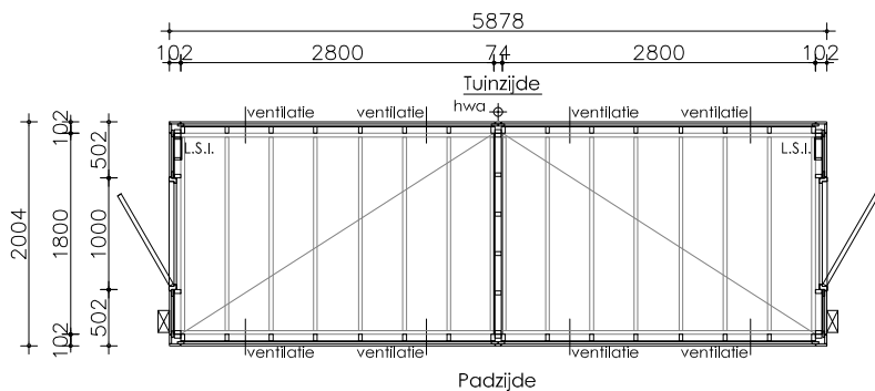
LCBU dubbele berging Type DLH: • Aantal getekend : 00 stuks
